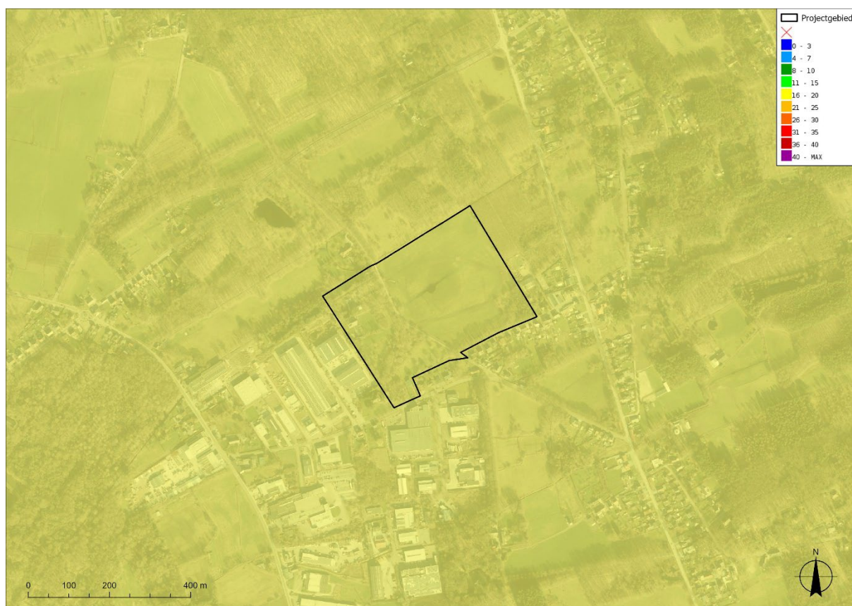
Figuur 41: Fijn stof - \text{PM}_{10} (jaargemiddelde 2022) met aanduiding van het plangebied
