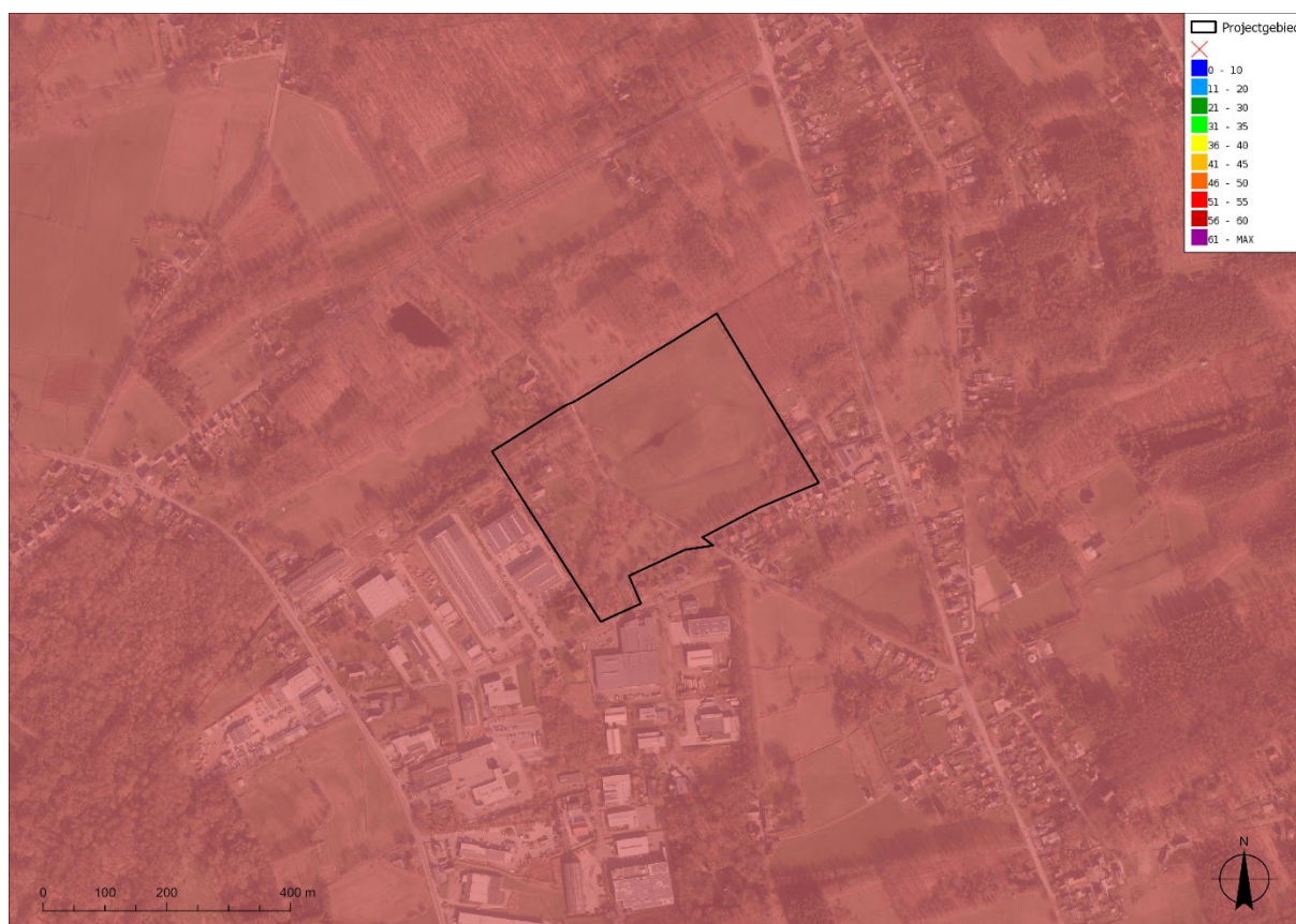
Figuur 43: O3 (jaargemiddelde 2022) met aanduiding van het plangebied
