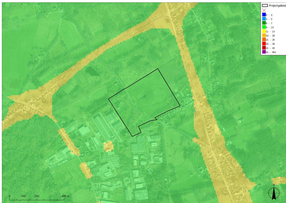
Figuur 40: Stikstofdioxide \text{NO}_2 (jaargemiddelde 2022) met aanduiding van het plangebied
